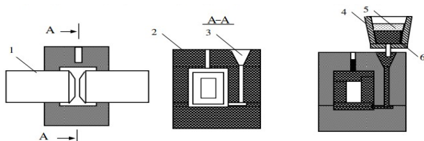
H.6.1. Sơ đồ hàn nhiệt nóng chảy
