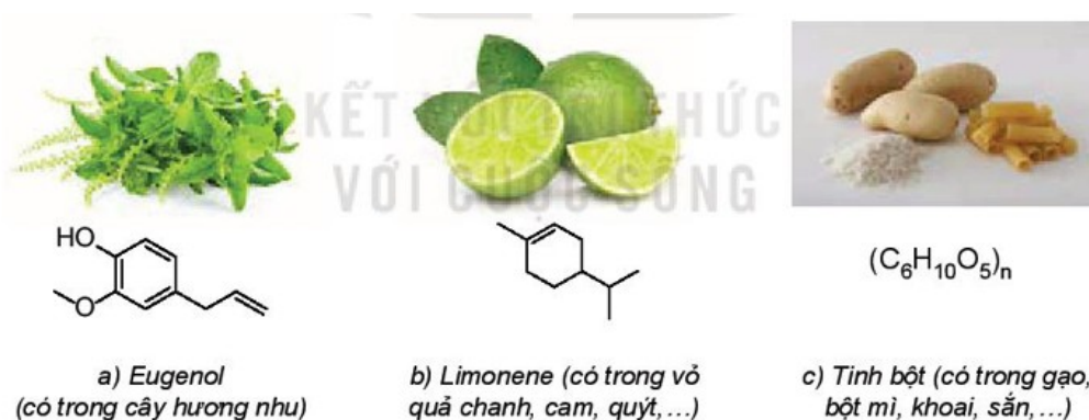
Hình 10.1. Một số hợp chất hữu cơ trong tự nhiên
