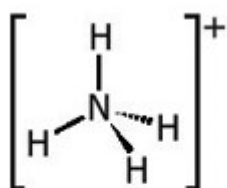
Hình 5.3. Dạng hình học của ion ammonium
