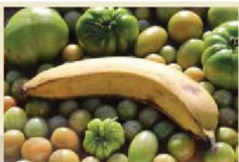
Hình 16.7. Khí ethylene sinh ra từ
