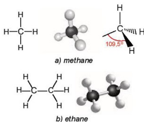
Hình 15.1. Công thức cấu tạo và mô hình phân tử của methane và ethane
