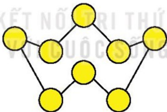
Hình 7.3. Phân tử sulfur \text{S}_8
